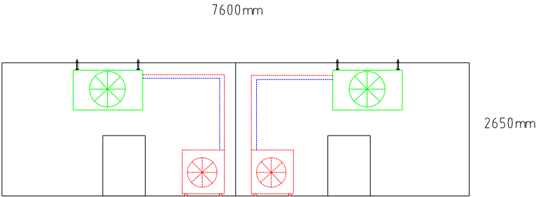
立面图
